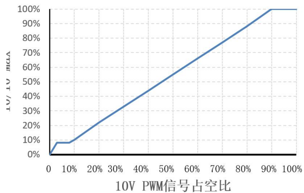
I_o/I_{oMax} VS 10V PWM
